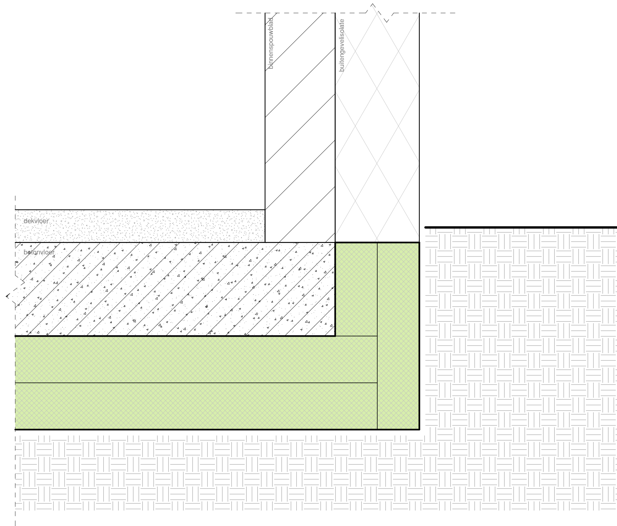
Buitengevelisolatie zonder vorstrand
